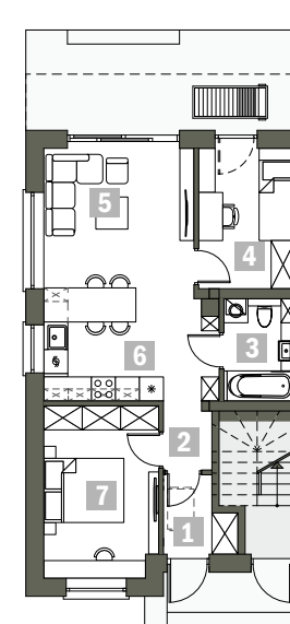
Rzut parteru
